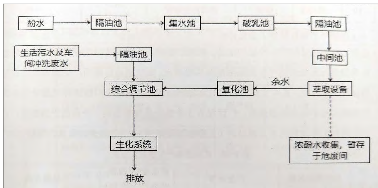
图 3-1 污水处理站工艺流程图
