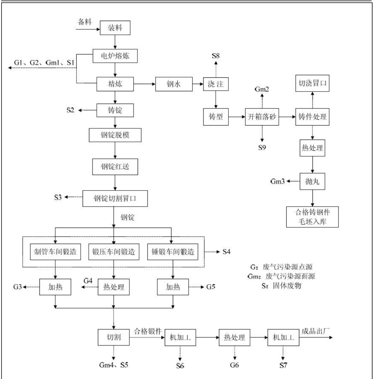
图 4-4 钢产品生产工艺流程及产污节点图
