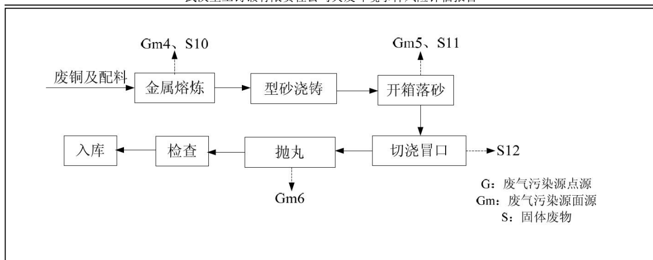
图 4-5 铜产品生产工艺流程及产污节点图
