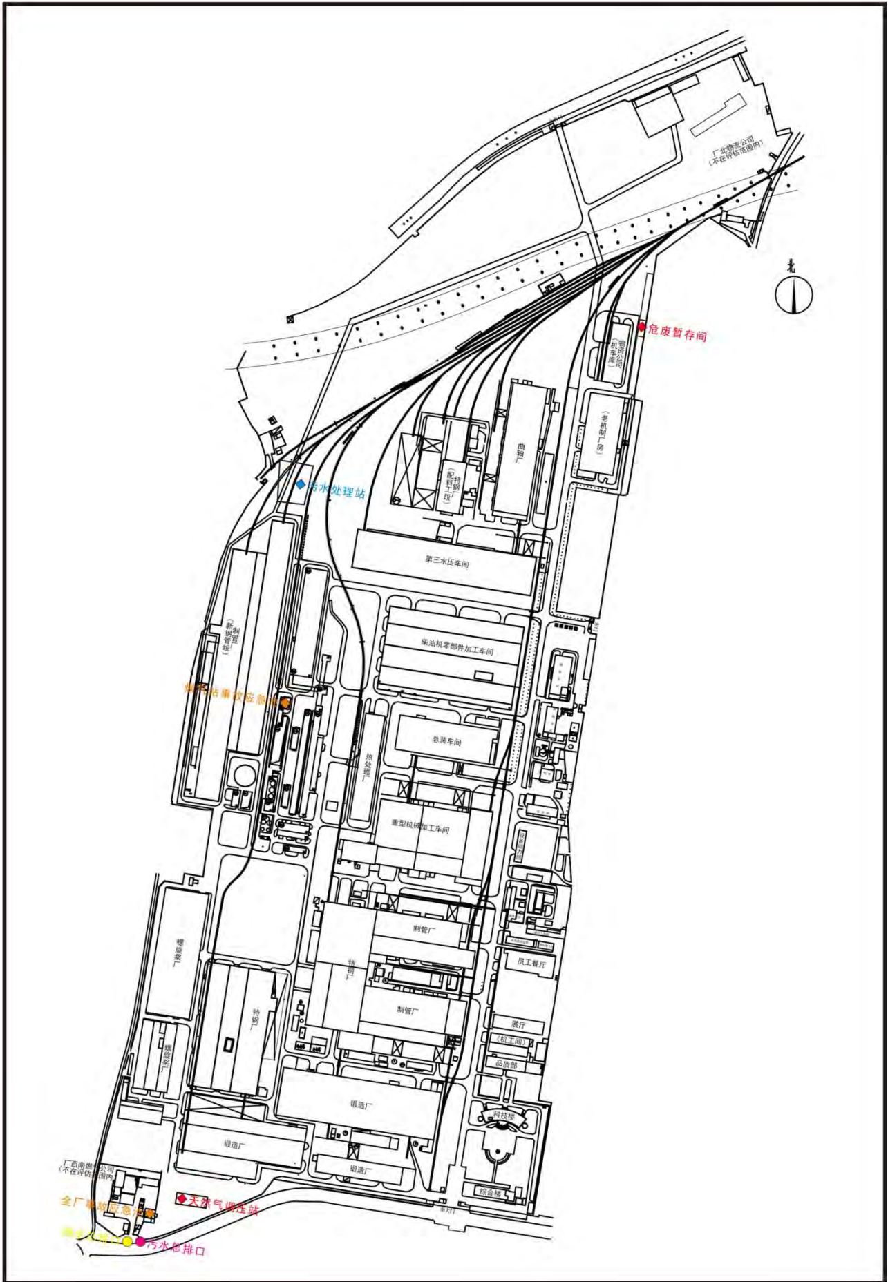
附图3 武汉重工铸锻有限责任公司厂区平面布置图
